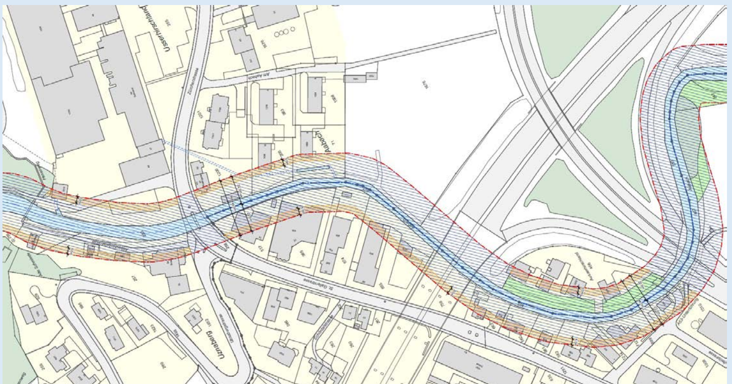
Auszug aus dem revidierten Sondernutzungsplan Gewässerraum Aabach
