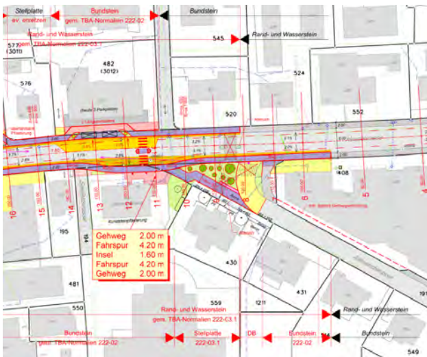
Planausschnitt 2
