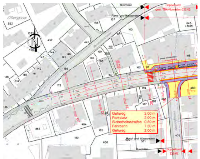
Planausschnitt 3
