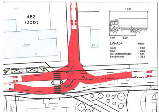
Zu- und Wegfahrt Sennhüttenstrasse
