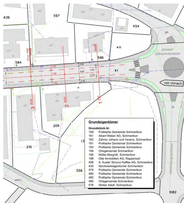
Plananschnitt 1
